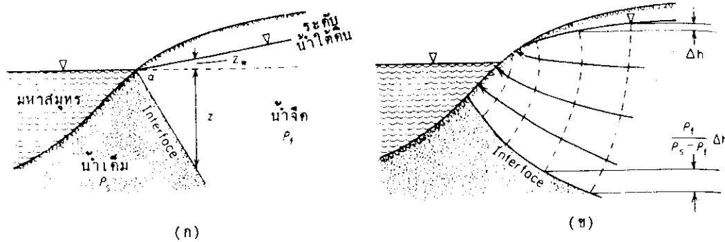
รูปที่ 6.9 แนวปะทะระหว่างน้ำเค็มกับน้ำจืด (saltwater-freshwater interface) ในชั้นหินอุ้มน้ำชายฝั่งที่ไม่ถูกกึ่งกัก (unconfined coastal aquifer)
