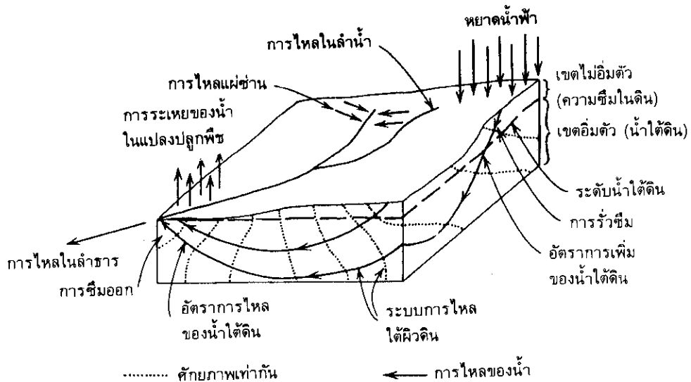
รูปที่ 6.1 แผนผังแสดงความสัมพันธ์ระหว่างอุทกวัฏจักรกับน้ำใต้ดิน
