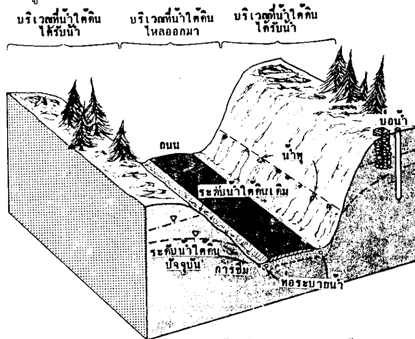
รูปที่ 6.7 ผลกระทบจากการตัดถนนผ่านชั้นหินอุ้มน้ำ ซึ่งจะทำให้ระดับน้ำใต้ดินลดลงอันเป็นสาเหตุทำให้บ่อน้ำแห้งและน้ำใต้ดินซึมลงมาบนถนน
