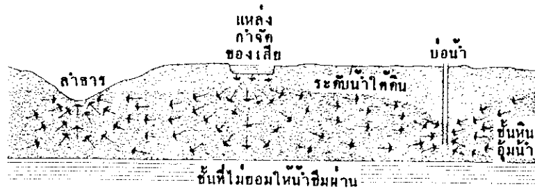
รูปที่ 6.10 การชะล้างจากแหล่งกักจัดของเสียสู่น้ำใต้ดิน และเคลื่อนที่เข้าไปยังบ่อน้ำ (ขวามือ) และลำธาร (ซ้ายมือ)
