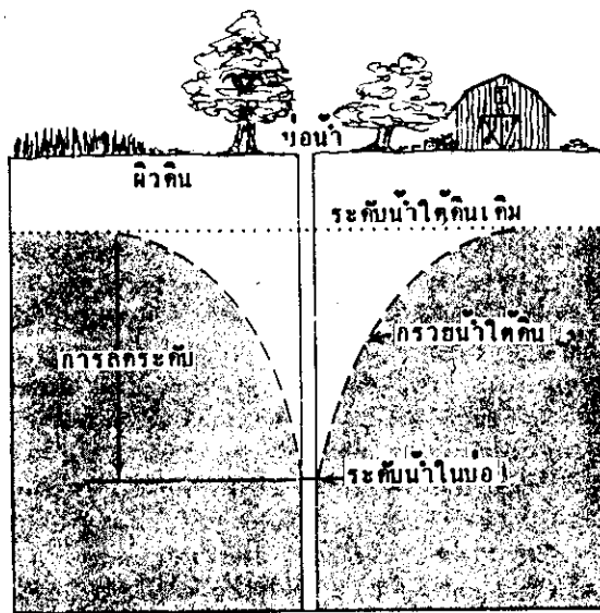
รูปที่ 6.5 การลดระดับ (drawdown) ของระดับน้ำใต้ดิน และกรวยน้ำใต้ดิน (cone of depression) ซึ่งเกิดจากการสูบน้ำจากบ่อ ขนาดของกรวยจะสัมพันธ์กับการสูบน้ำและการขบขี้มน้ำได้ของชั้นหินอุ้มน้ำ
