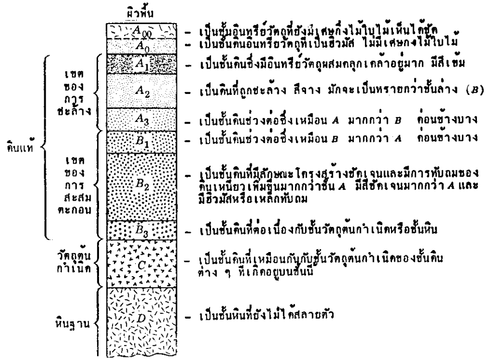
รูปที่ 5.2 ตัวอย่างหน้าตัดดินซึ่งแสดงชั้นดินต่าง ๆ ทุกชนิด ที่มา : Strahler, 1975.
