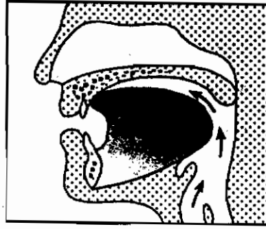
/tʃ/, /dʒ/
