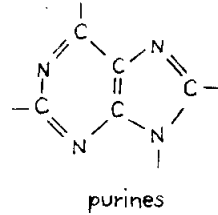
ภาพ 3-1 แสดงสูตรโครงสร้างของสารอินทรีย์ทั้งหมด
