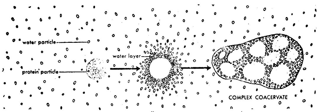
ภาพ 3-4 แสดงลำดับขั้นของสมมติฐานโคลออยด์เซอร์เวท
